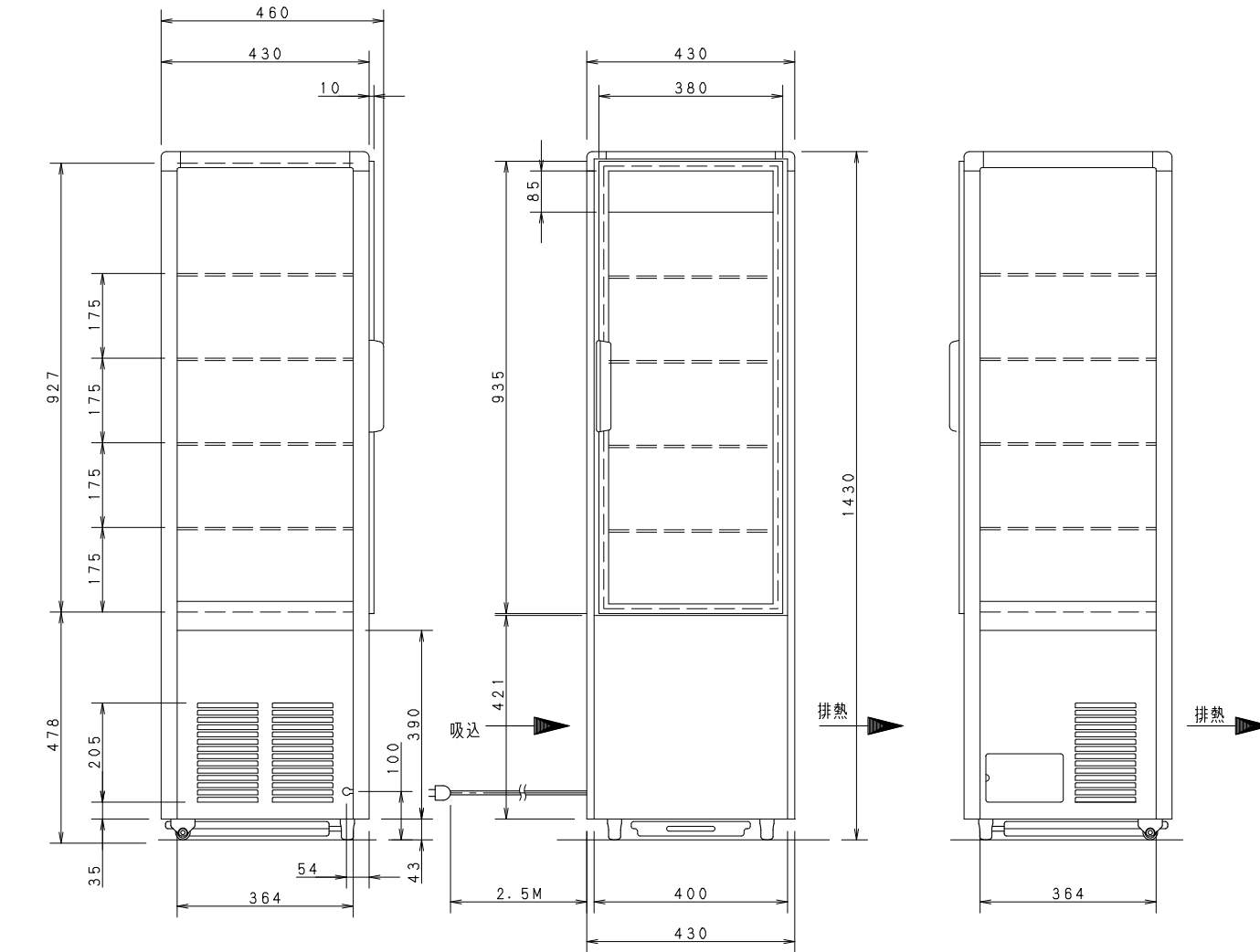
陳列部寸法
