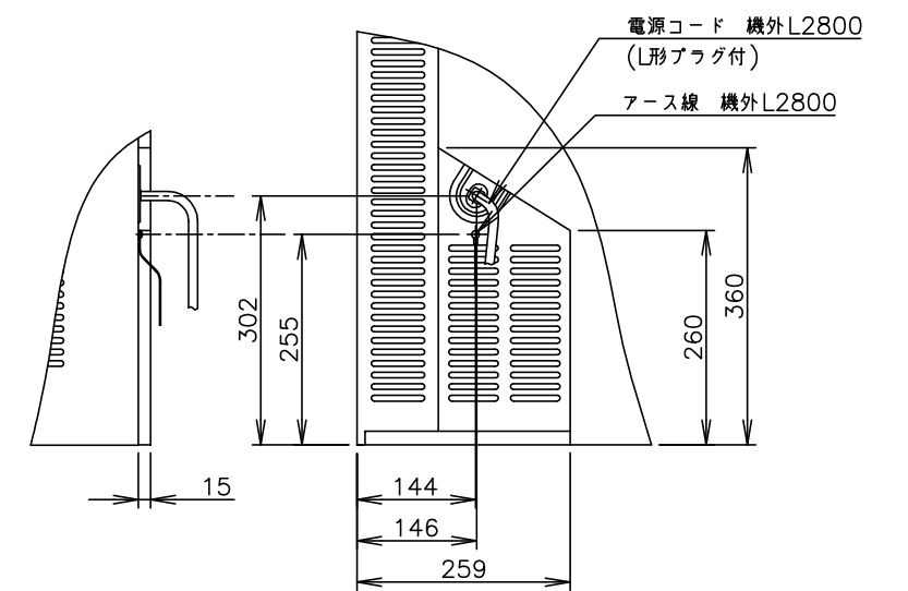
A矢视图 (1/10)
