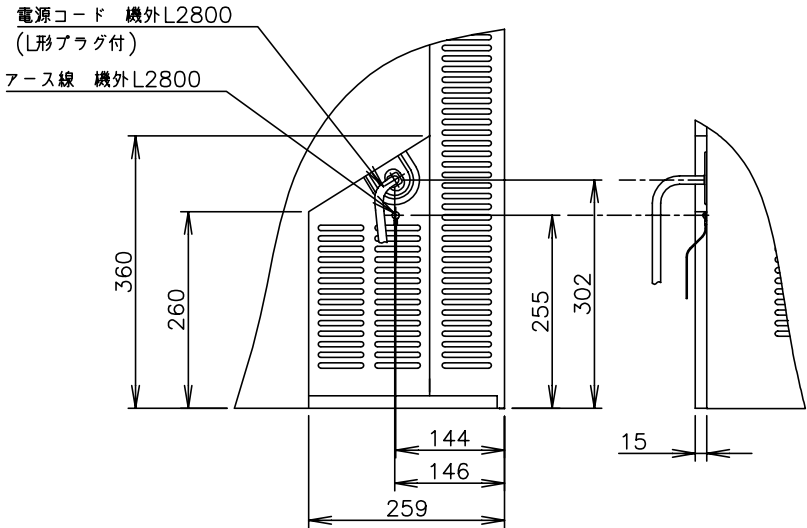
A矢视图(1/10)
