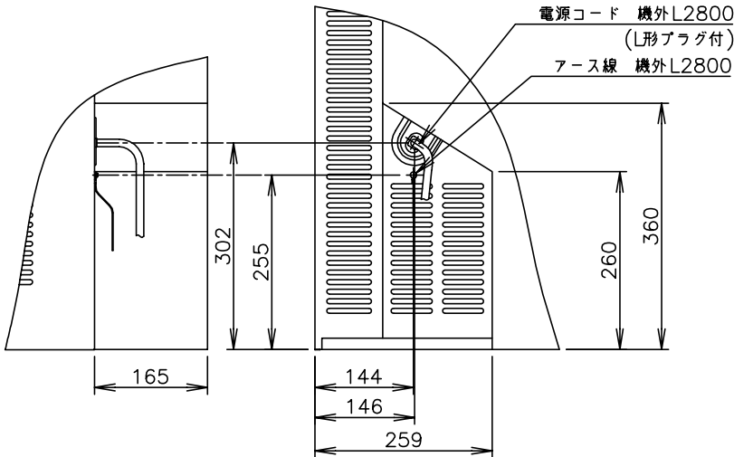
A矢视图 (1/10)
