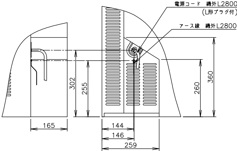
B矢视图 (1/10)
