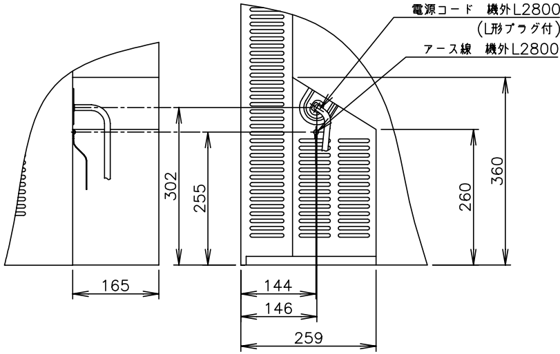
B矢視図 (1/10)
