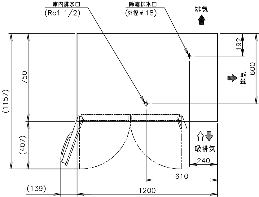
B矢視図 (1/10)
