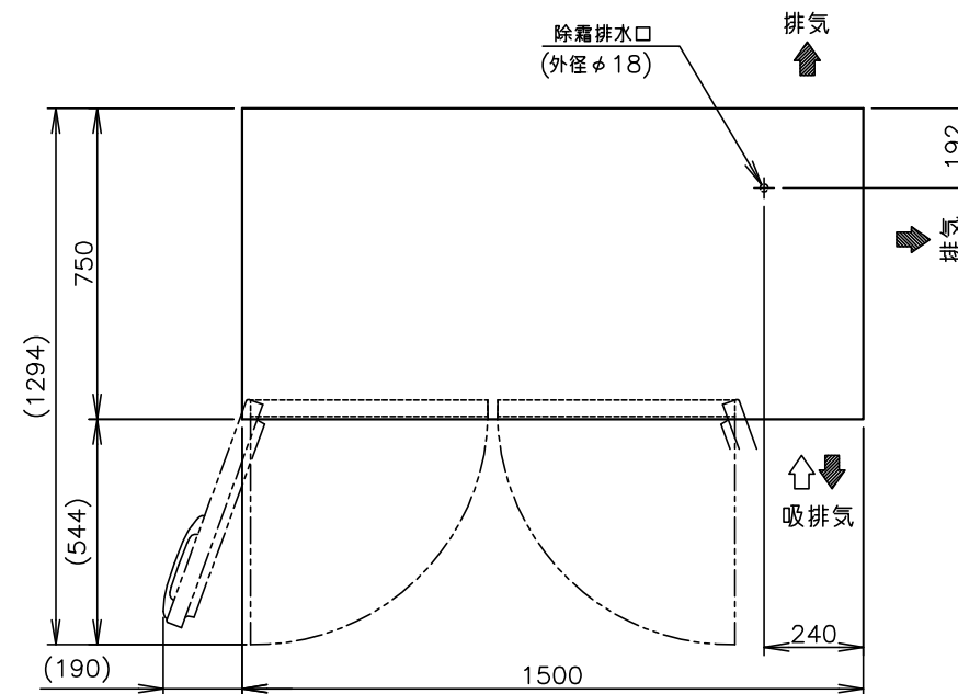
B矢视图(1/10)
