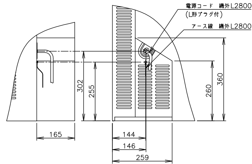
B矢视图(1/10)
