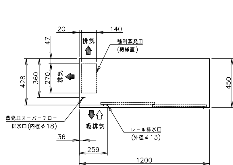
A矢视图(1/10)
