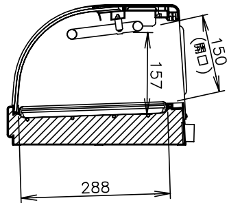
側面断面図
