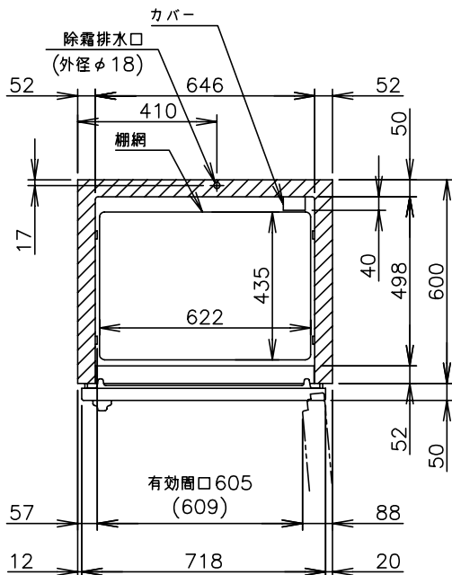
平面断面図(上室)
