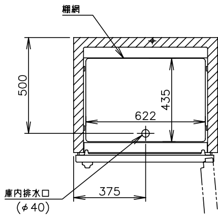
平面断面図(下室)
