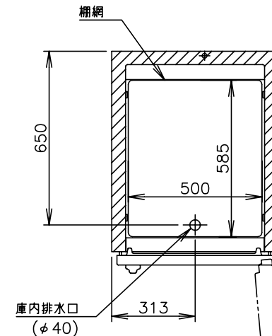
平面断面图(下室)
